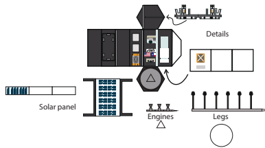
MAPP rover
